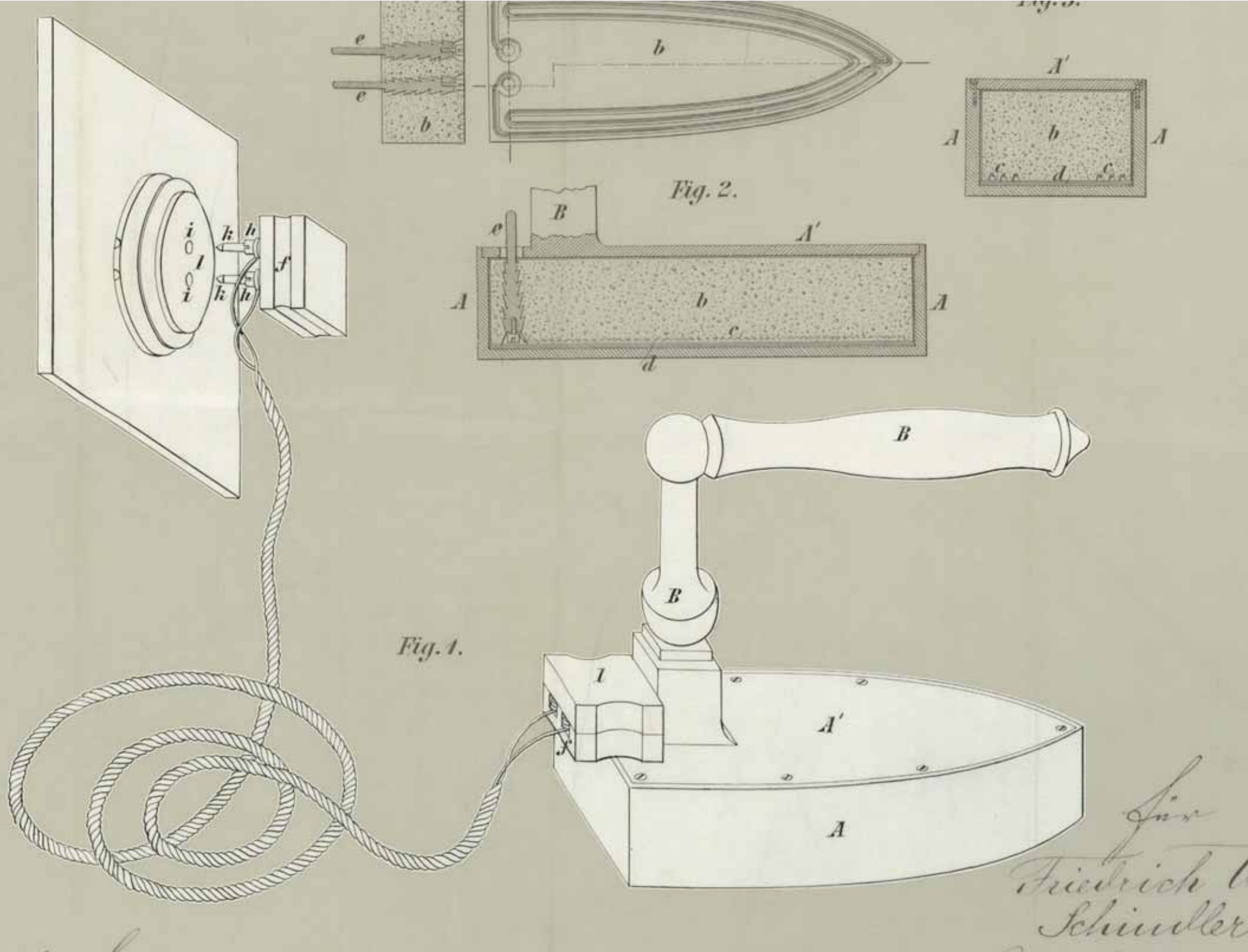
Patentvorläufer für ein elektrisches Bügeleisen des Kennelbacher Strompioniers Friedrich Wilhelm Schindler, 1893.
